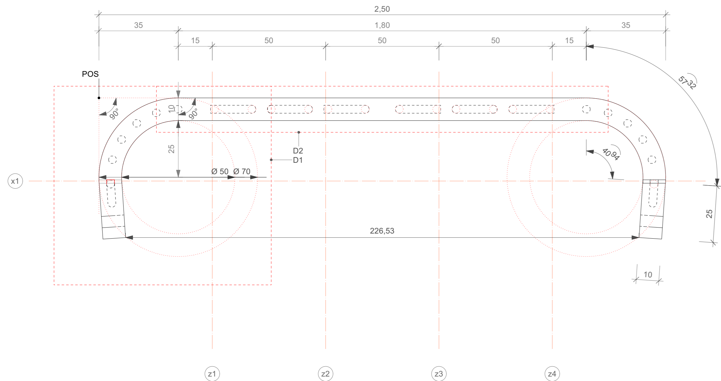
Übersicht A (o) M 1:10
